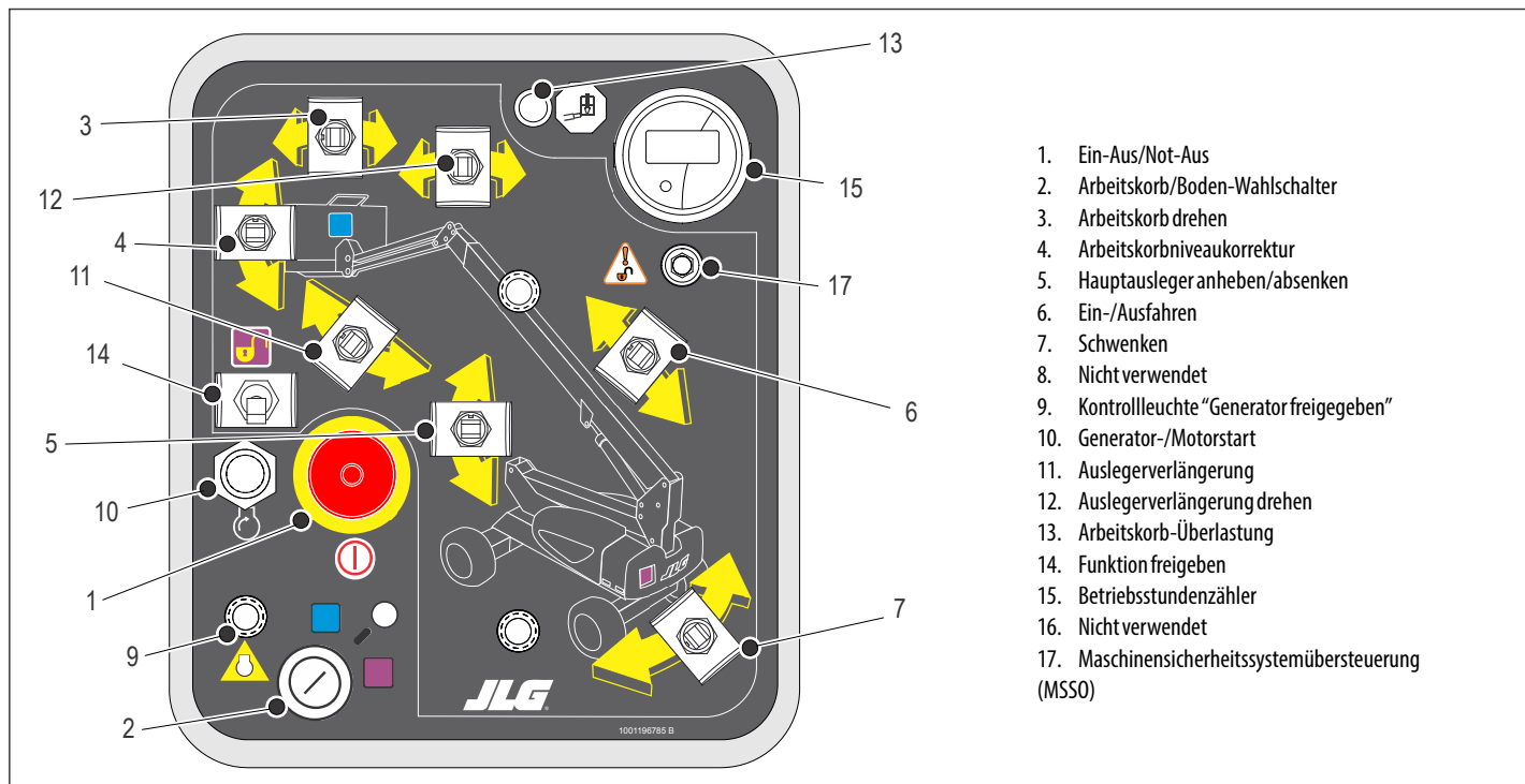
Abbildung 3-4. Boden-Bedienpult mit Maschinensicherheitssystemübersteuerung (MSSO) (nur CE) – Ser.nr. 0300202137 bis jetzt
