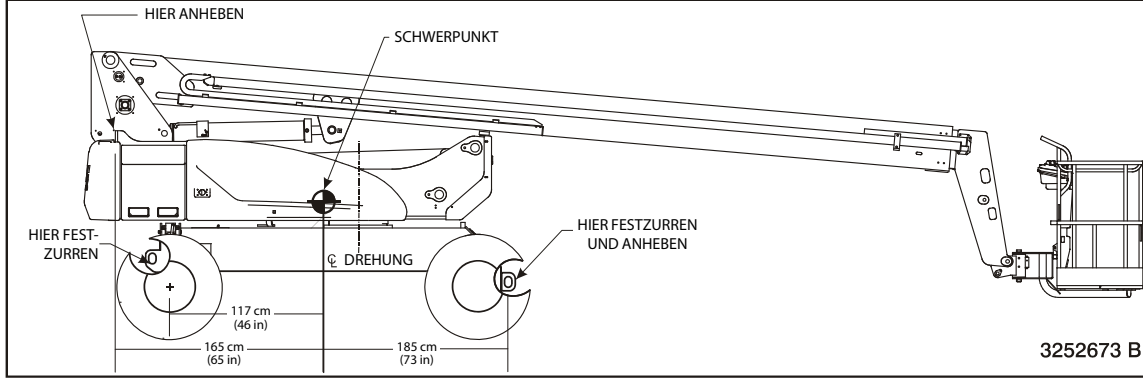
Abbildung 4-5. Anhub- und Festzurrdiagramm
