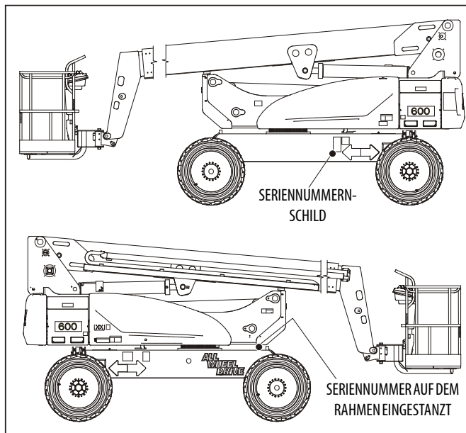
Abbildung 6-1. Anbringungsorte der Seriennummer
