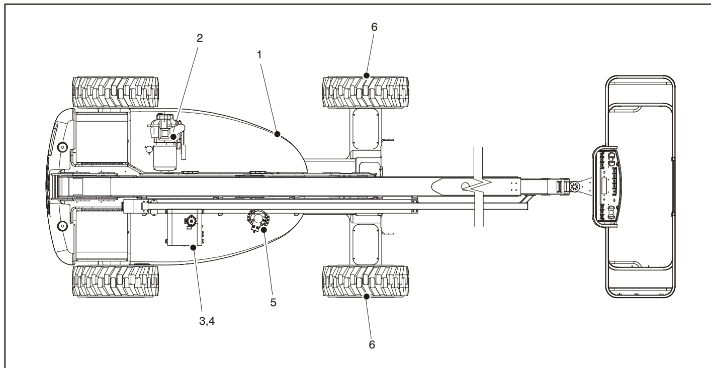
Abbildung 6-2. Wartung durch das Bedienungspersonal und Abbildung der Schmierpunkte
