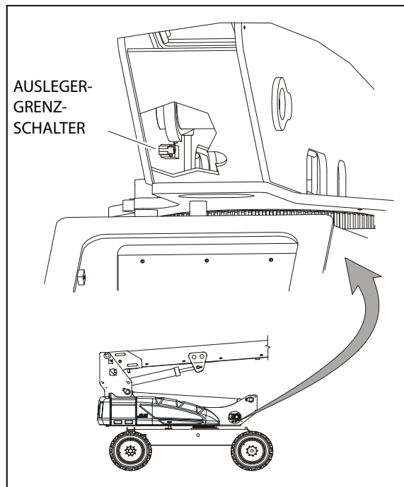
Abbildung 2-6. Tägliche Sichtkontrolle – Blatt 3 von 4
