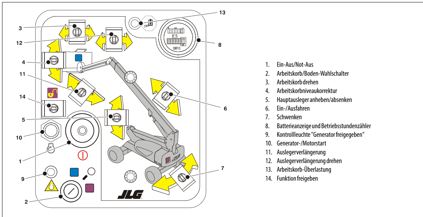
Abbildung 3-2. Boden-Bedienpult mit Funktionsfreigabe
