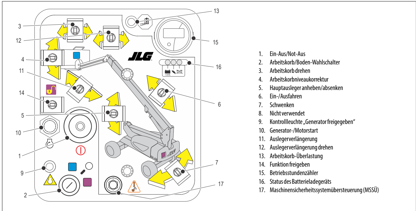
Abbildung 3-3. Boden-Bedienpult mit Maschinensicherheitssystemübersteuerung (MSSÜ) – nur CE – vor Ser.nr. 0300202137
