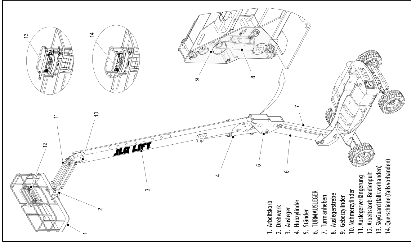
Abbildung 2-3. Grundlegende Bezeichnungen – Blatt 3 von 3
