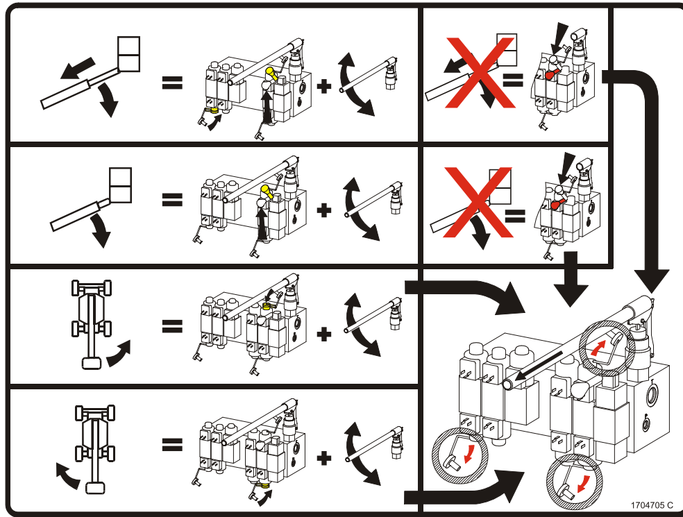
Abbildung 5-1. Aufkleber für manuelles Absenken
