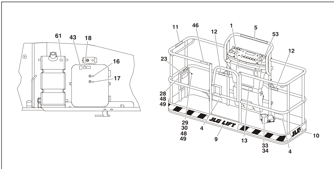
Abbildung 4-8. Aufkleberanordnung - Blatt 3 von 4
