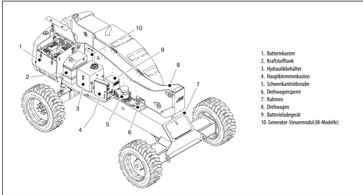
Abbildung 2-1. Grundlegende Bezeichnungen – Blatt 1 von 3
