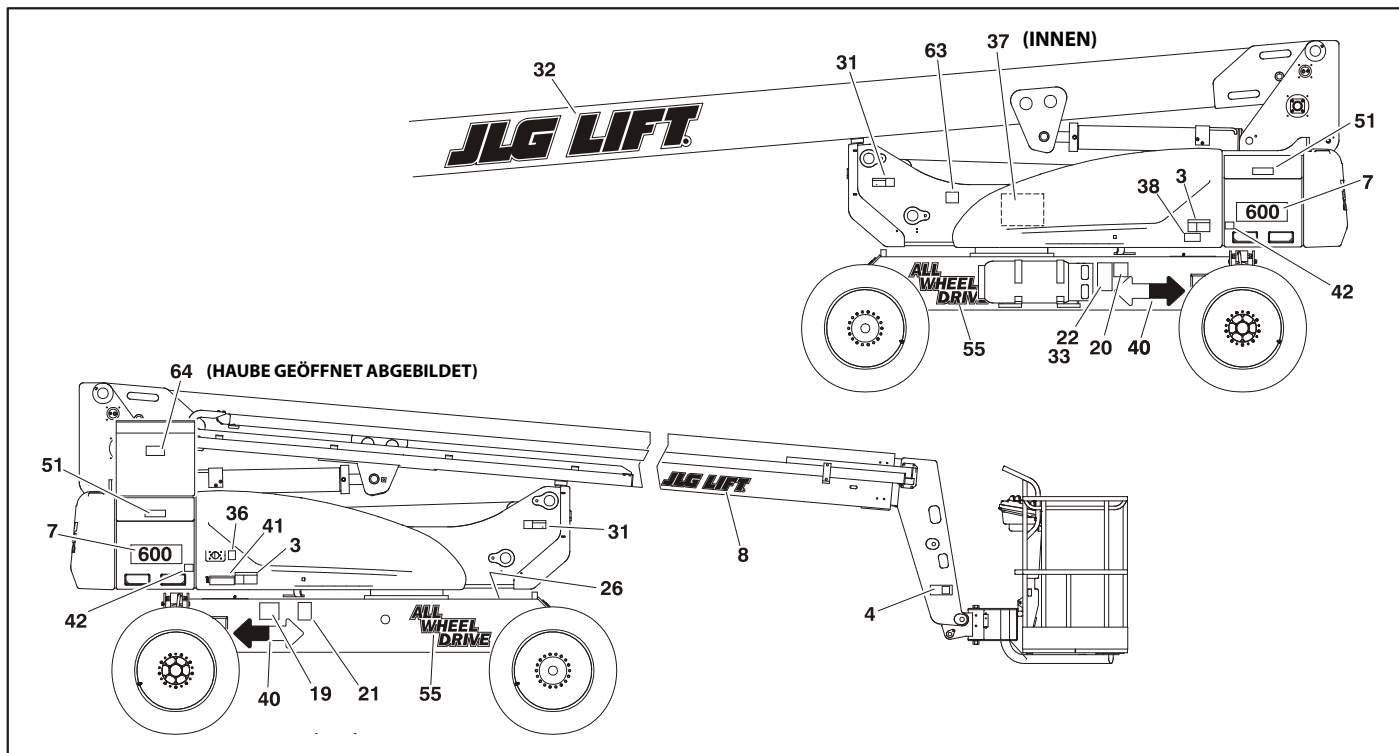
Abbildung 4-6. Aufkleberanordnung – Blatt 1 von 4
