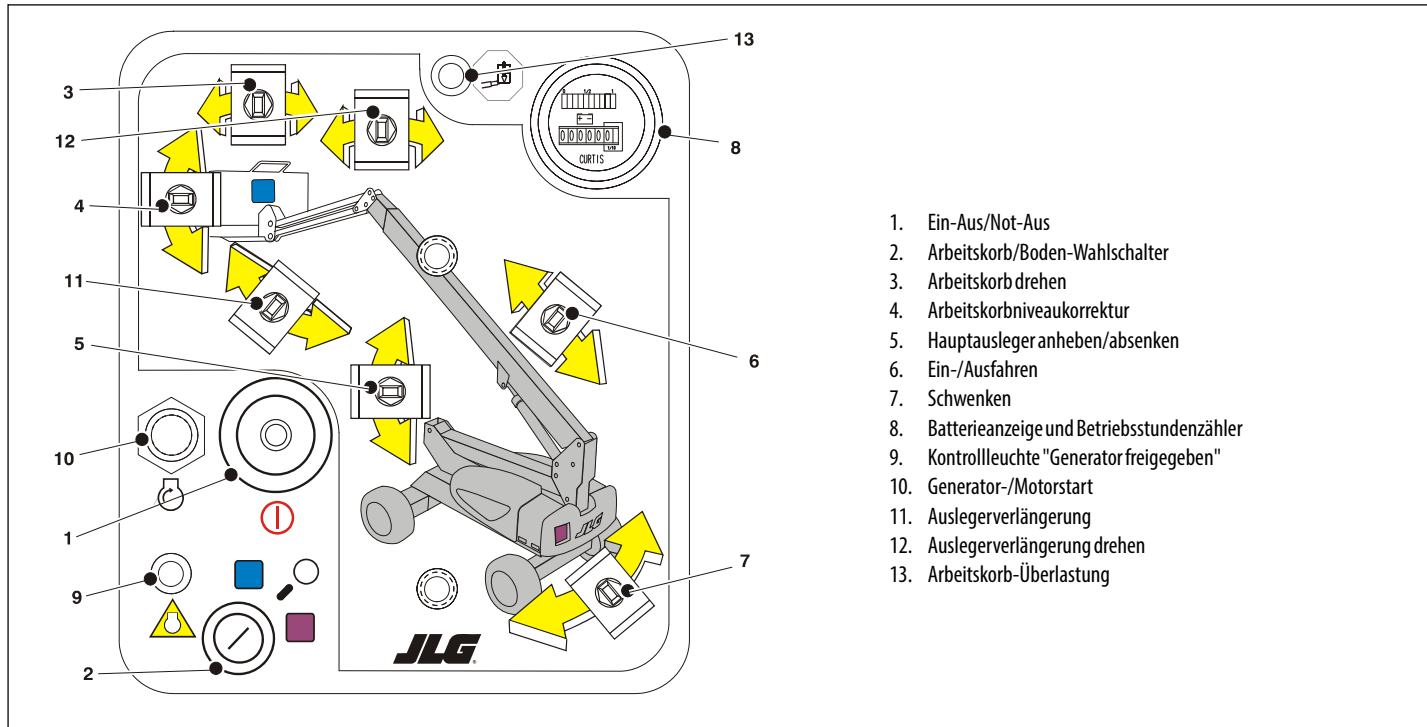
Abbildung 3-1. Boden-Bedienpult
