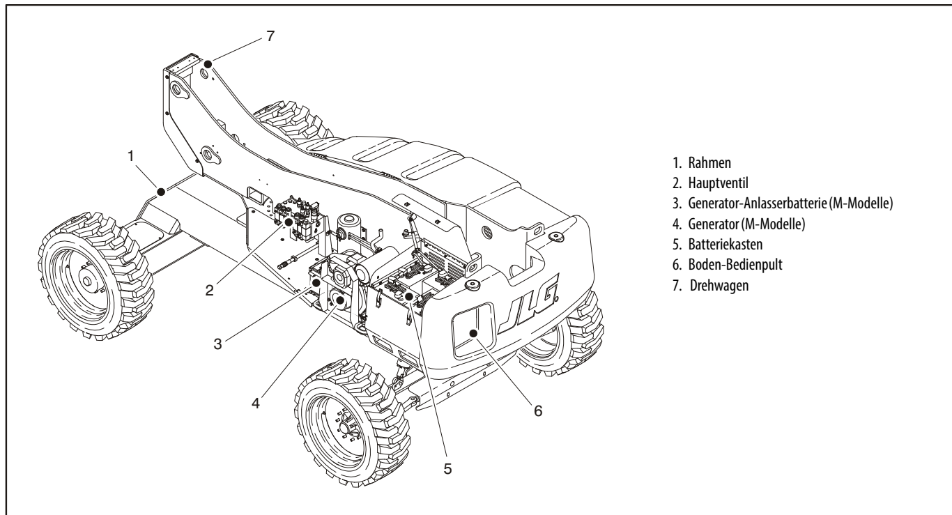
Abbildung 2-2. Grundlegende Bezeichnungen – Blatt 2 von 3
