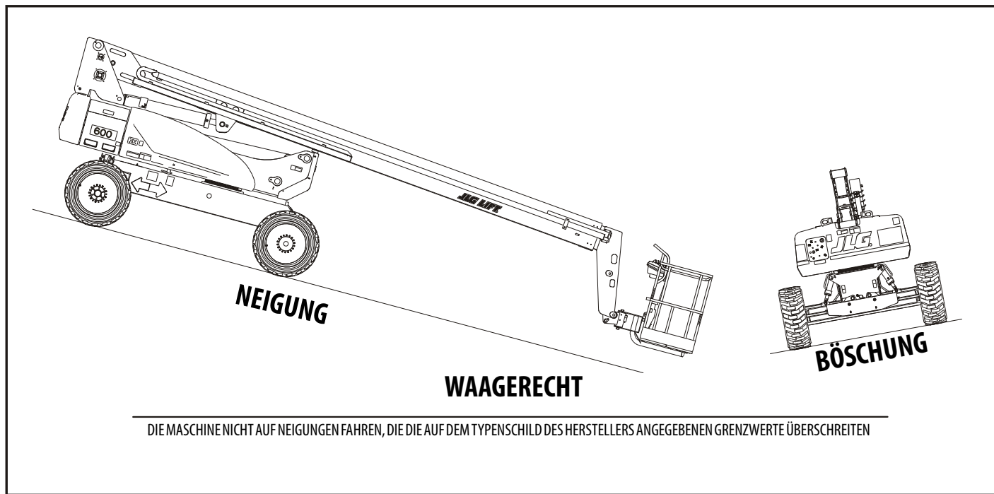
Abbildung 4-3. Neigung und Böschungen
