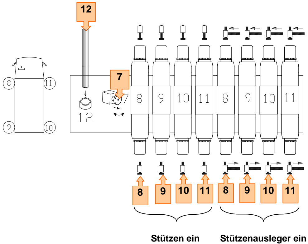
Stützensteuerblock am Fahrzeugheck links
