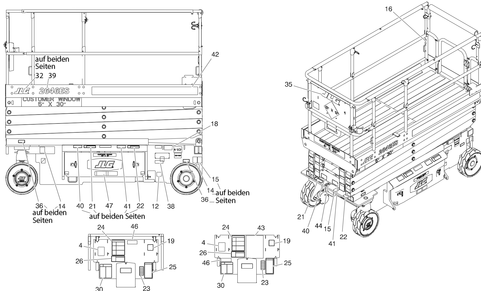
Abbildung 5-8. Aufkleberanordnung - 2646ES und 3246ES - Blatt 1 von 2
