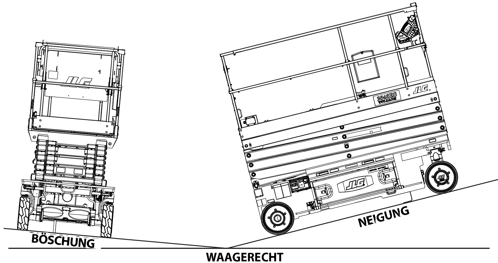
Abbildung 3-5. Neigung und Böschung – Fahren – Arbeitskorb verstaут
