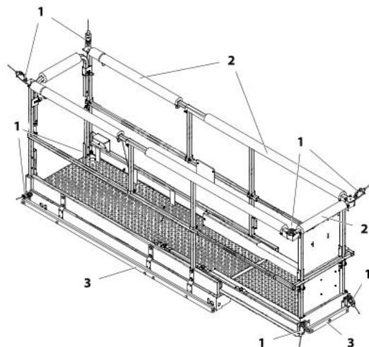
Abbildung 3-6. Soft-Touch-System
