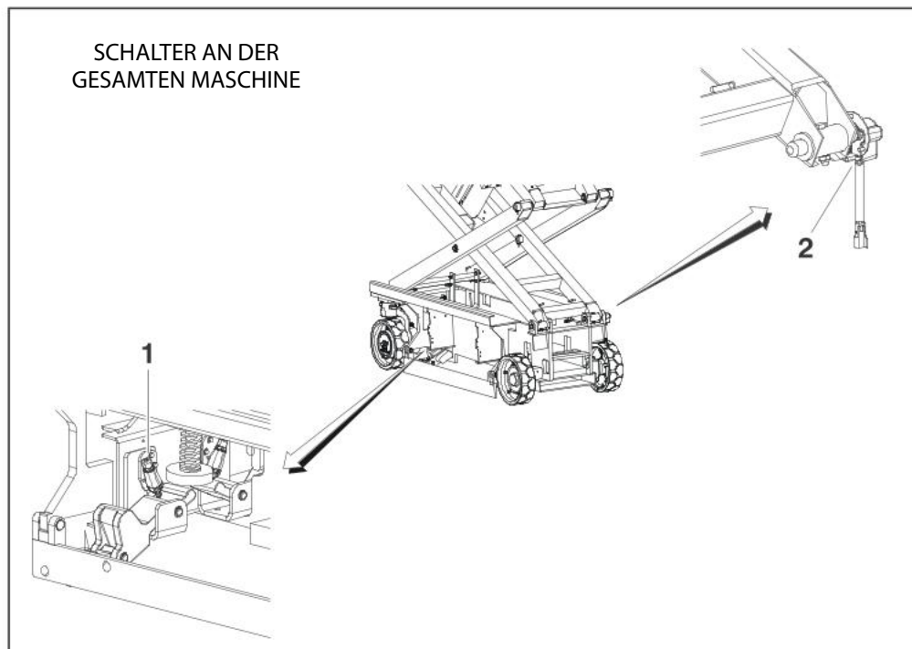
Abbildung 2-3. Schalieranordnung
