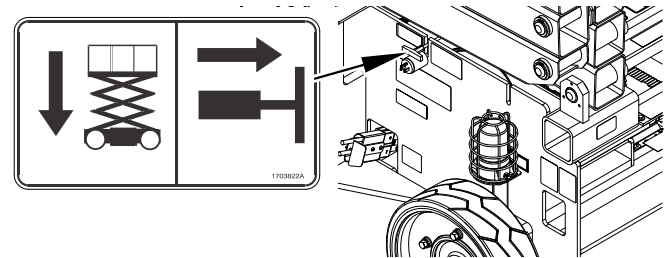
Manuelles Absenksystem - T-Griff-Anordnung
