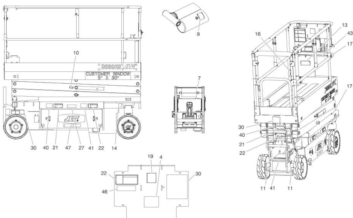
Abbildung 5-7. Aufkleberanordnung – 2032ES und 2632ES – Blatt 2 von 2
