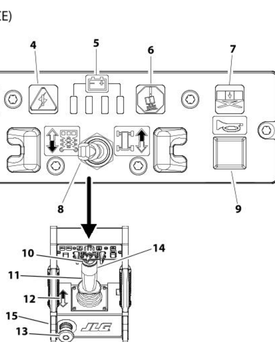
Abbildung 3-4. Arbeitskorb-Bedienpult
