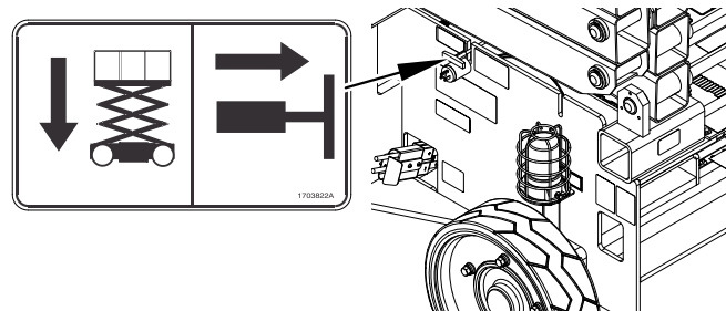
Manuelles Absenksystem – T-Griff-Anordnung
