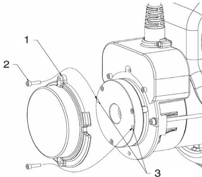
Abbildung 3-12. Manuelles Ausrücken
