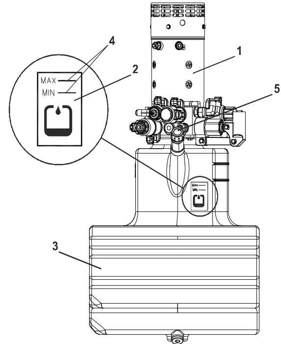
Bild 5-9. Hydraulikölkontrolle
