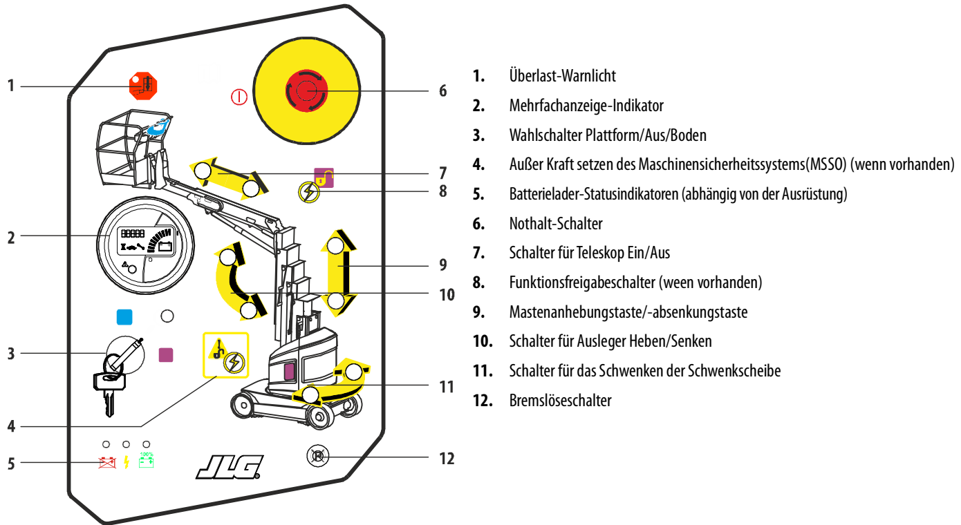
Bild 3-4. Boden-Steuerungsstation
