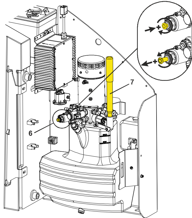
Bild 3-8. Manuelle Schwenkvorrichtung
