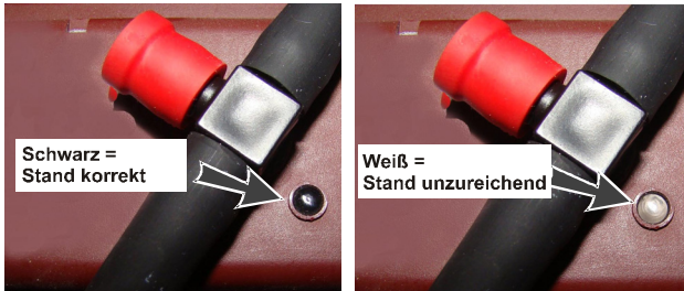
Bild 5-5. kontrolleuchte
