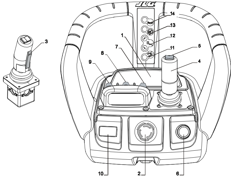
Bild 3-10. Plattform Steuerstation
