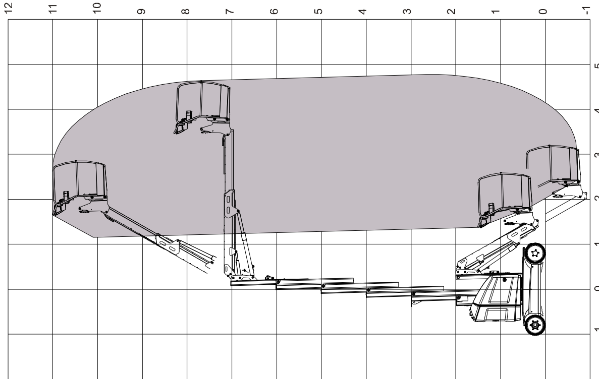
Bild 5-1. Bereichsdiagramm 12E/32E
