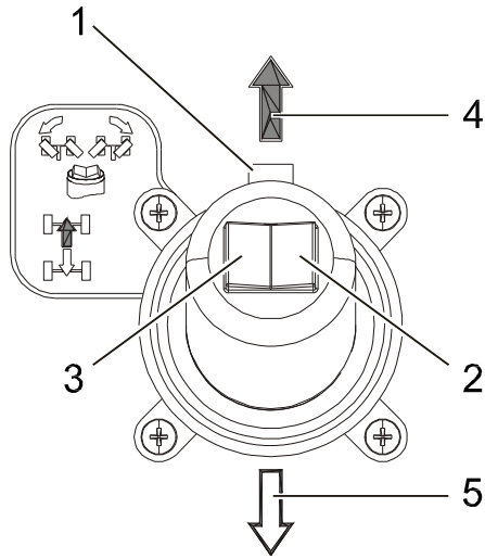
Bild 3-13. Lenk-/Fahrbedienelemente
