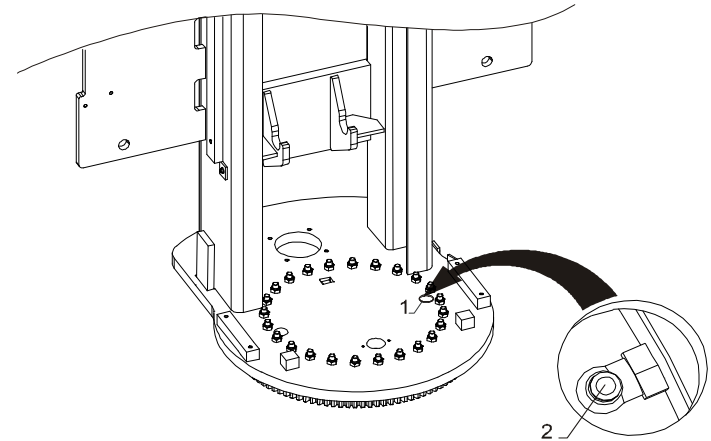
Bild 5-15. Schwenklagerungsschmierung
