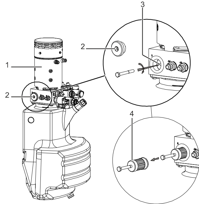
Bild 5-10. Ersetzen des Hydraulikfilters
