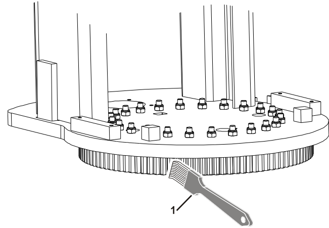
Bild 5-16. Schmierung der Schwenklagerungszähne
