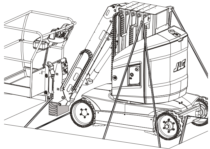
Bild 3-15. Festbinden der Maschine
