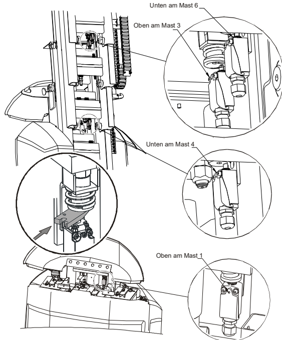
Bild 5-19. Schmierung der Kettensensor
