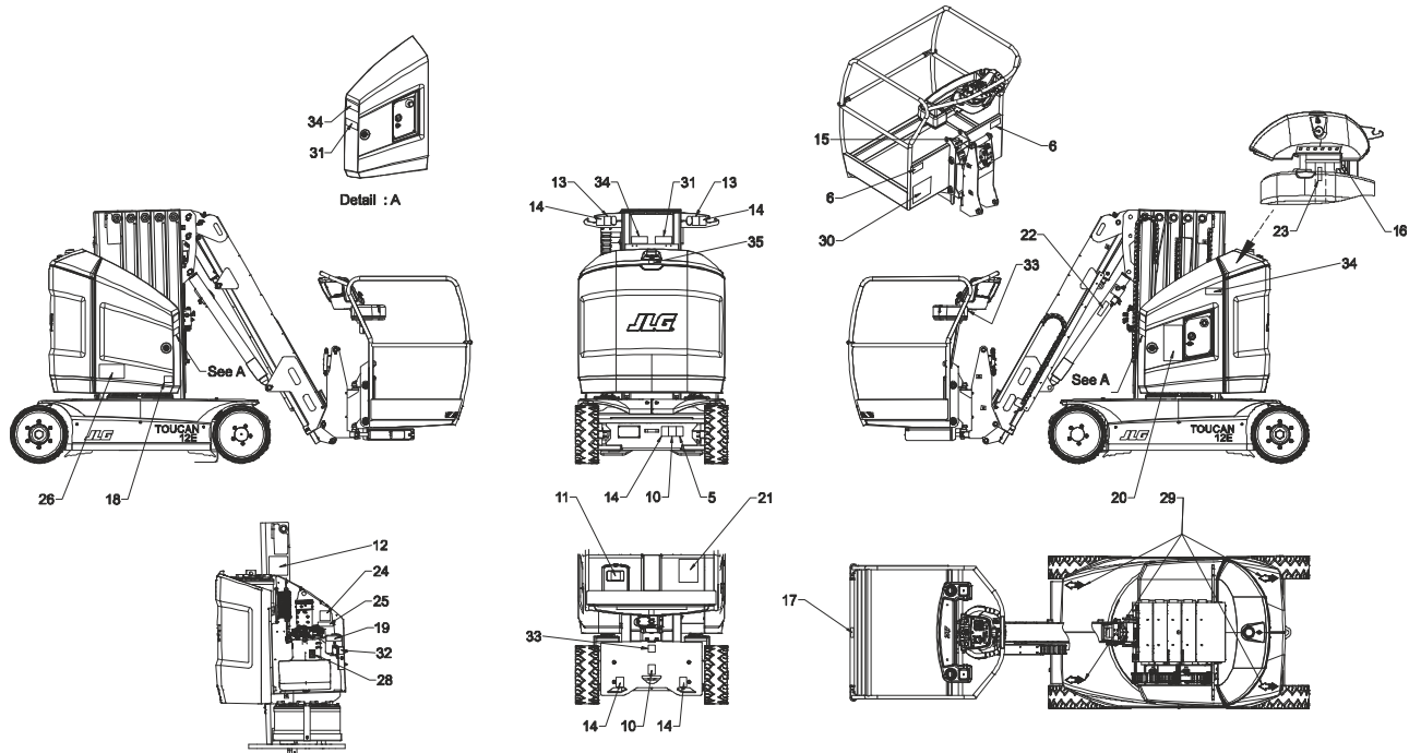
Figure 5-12. Anbringung der Maschinenaufkleber - Alle Märkte
