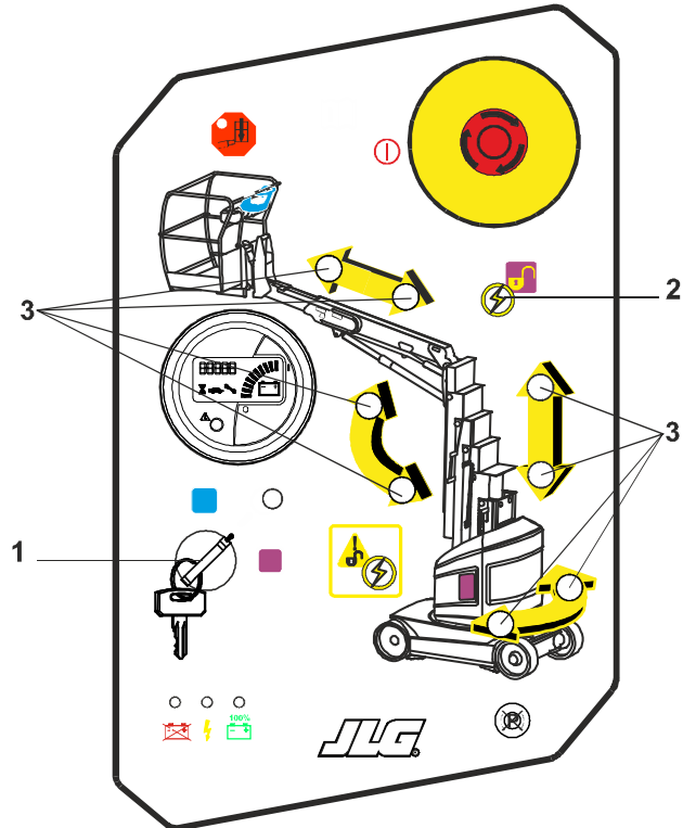
Bild 4-1. Notsteuerungen
