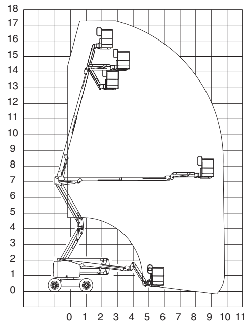
Z-51/30 Reichweitentabelle
