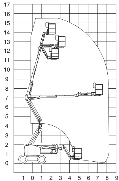
Z-45/25J Reichweitentabelle
